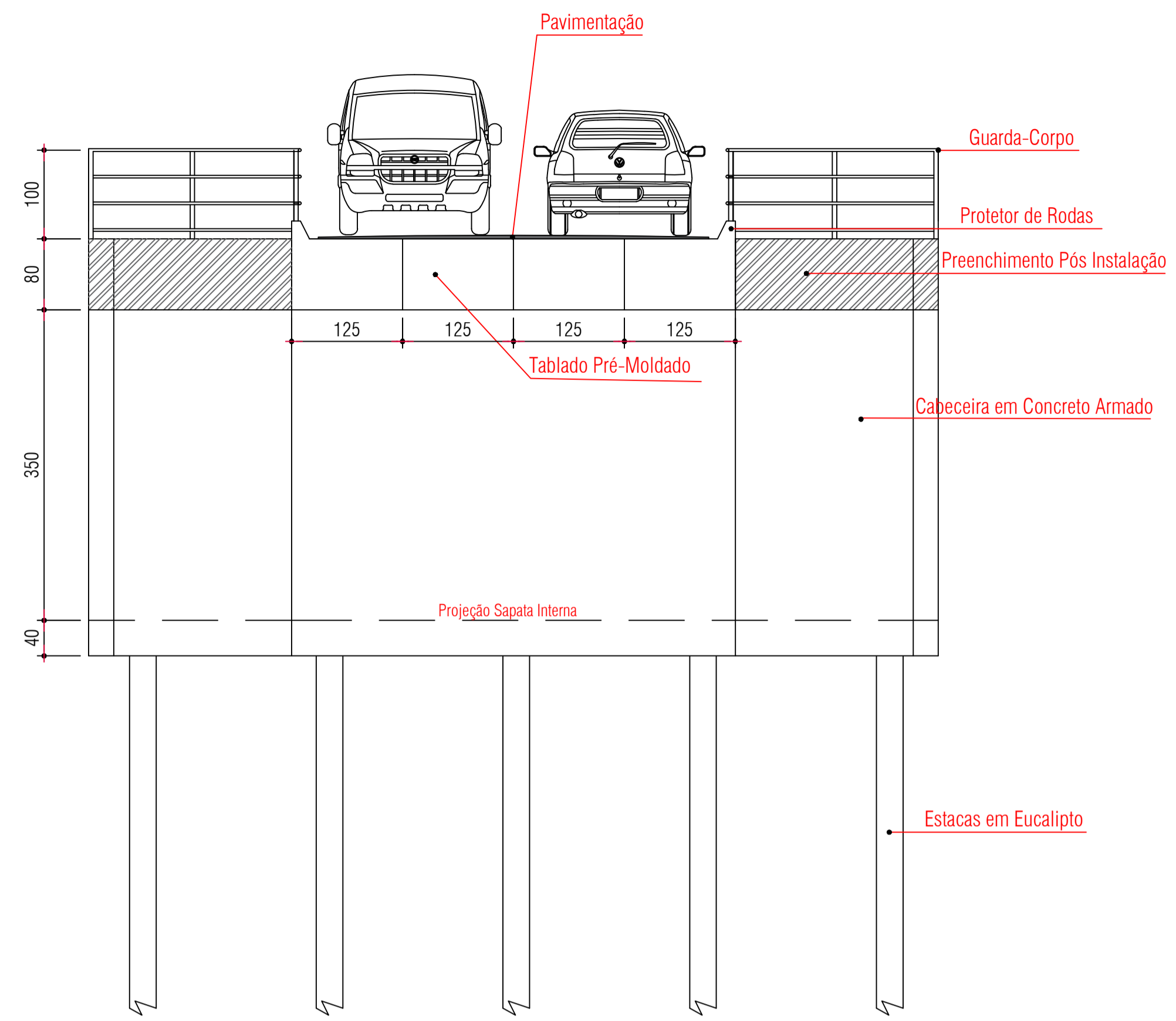
Corte Transversal Esc. 1:50
