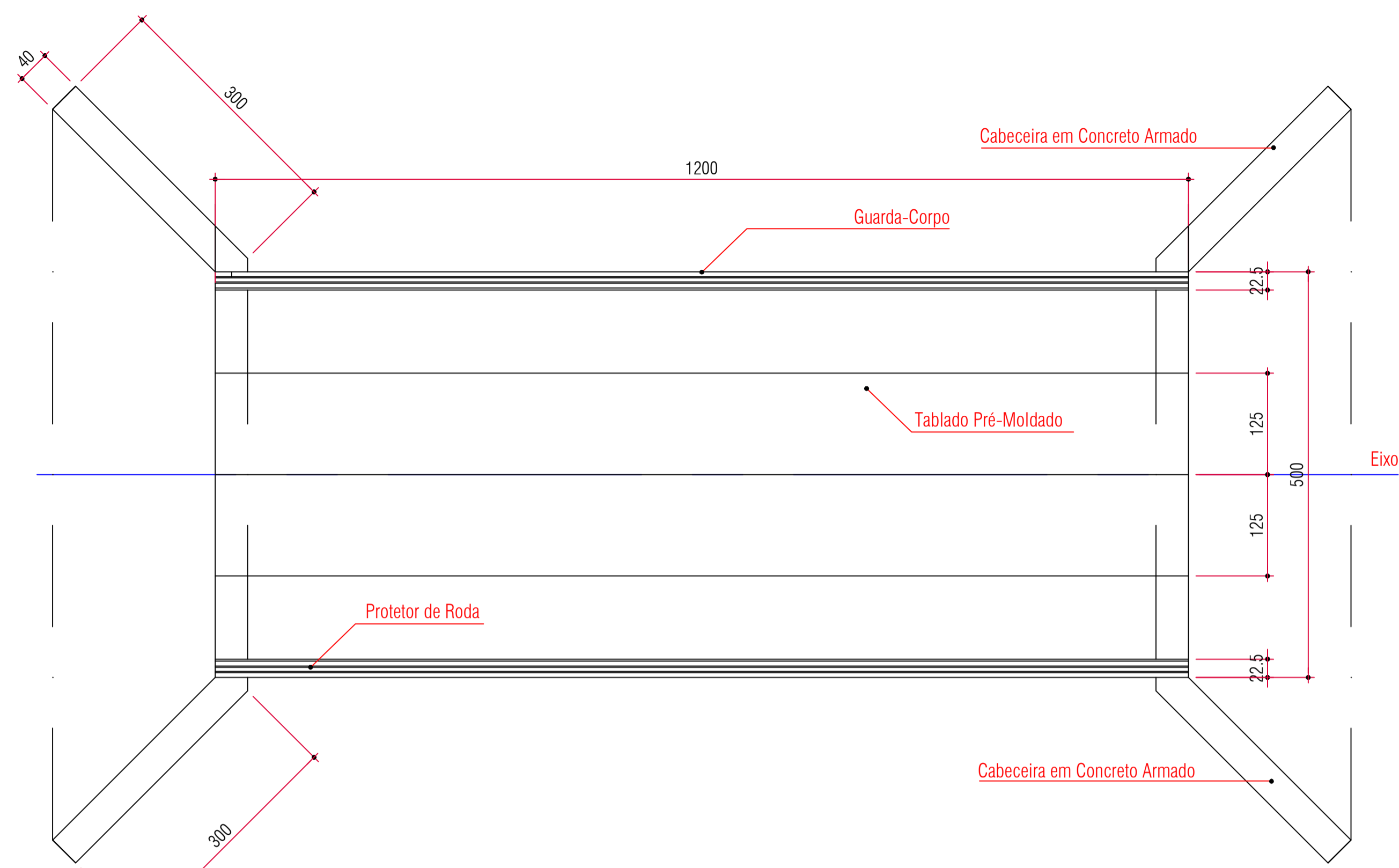
Vista Superior Esc. 1:50
